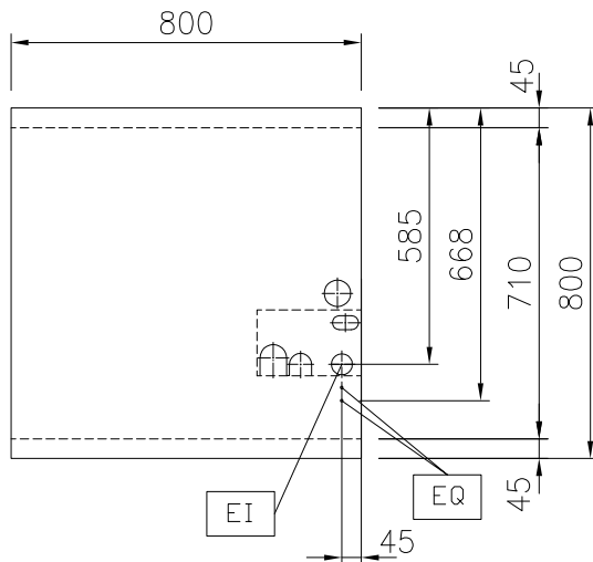
Boven aanzicht
