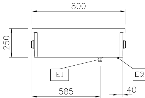
Zij aanzicht
